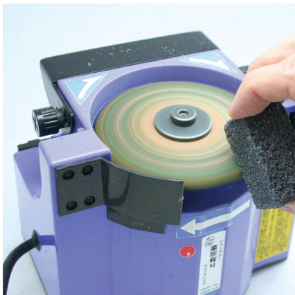
③面直しストーンを 皮バフのエッジにも 押し当てます
